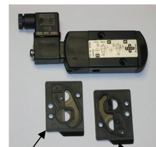
5/2 FUNKTION
